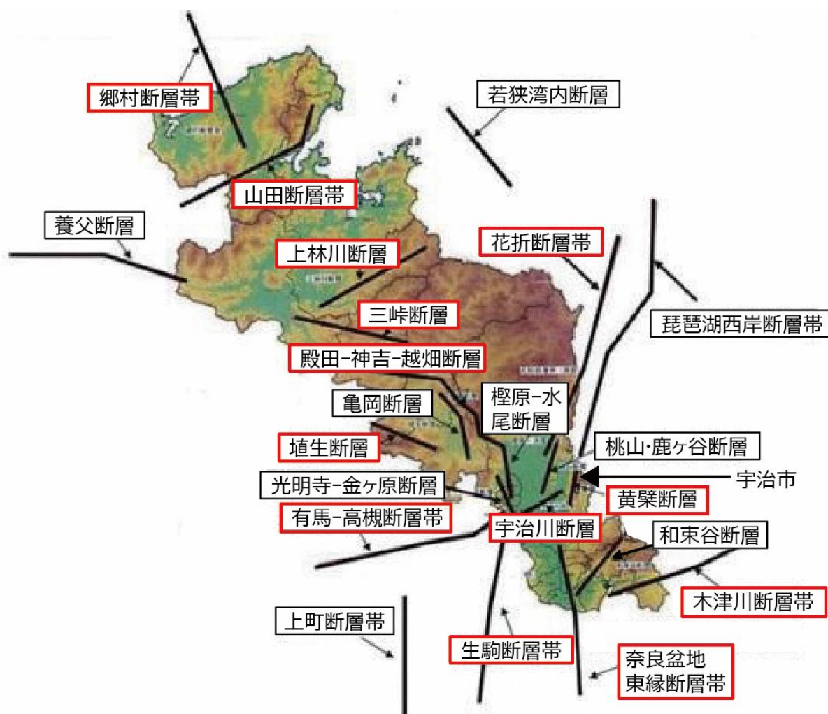
図8:断層分布図
