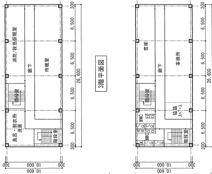
3階平面図
